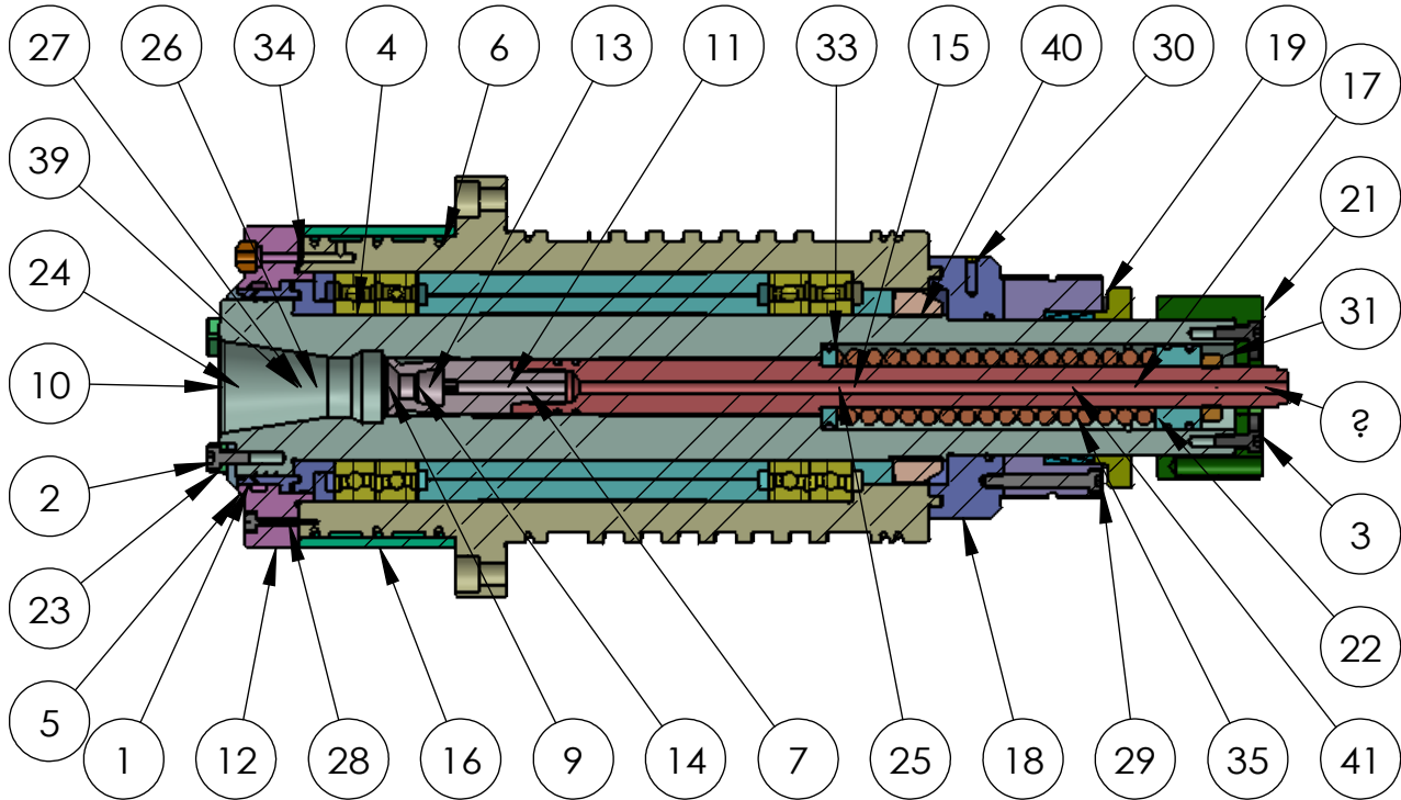
剖面圖 A-A
